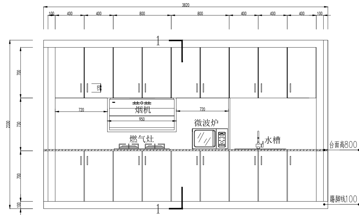
立面图（柜门关闭） 1:30
