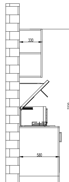
剖面图-从左侧看（1-1） 1:30
