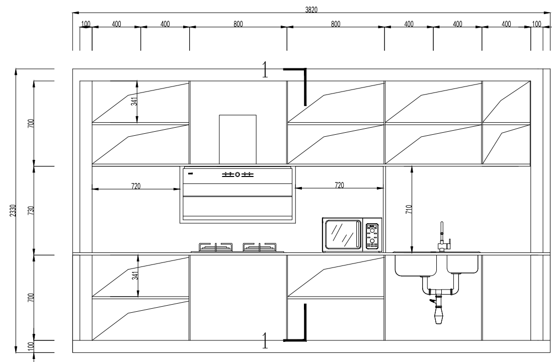
结构图（柜门打开） 1:30
