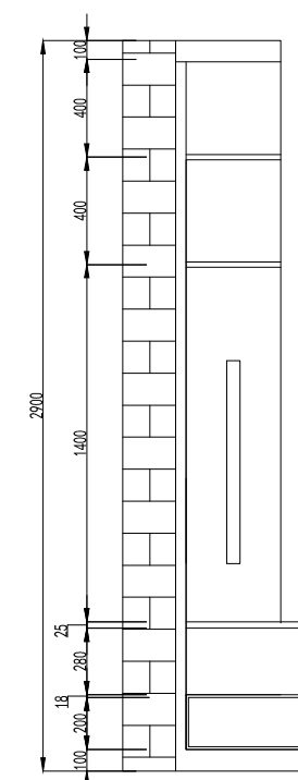
剖面图-从左侧看（1-1） 1:30
